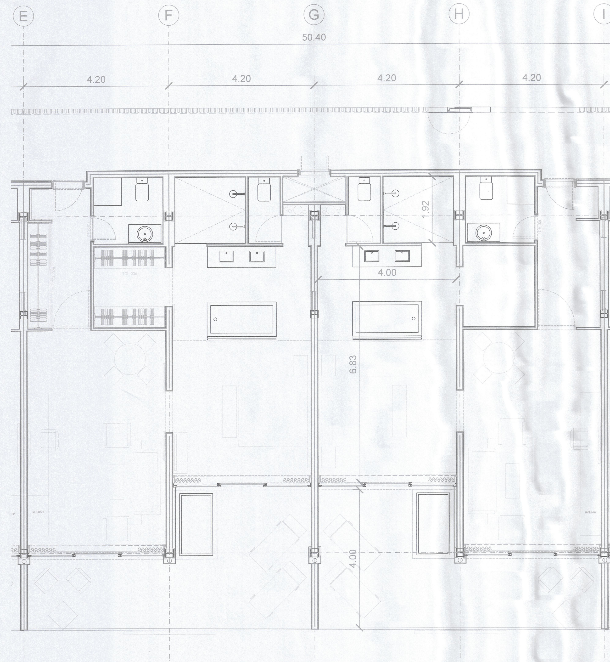
1 PLANTA HABITACION PREFERED ARQ-08 ESCALA 1:50
